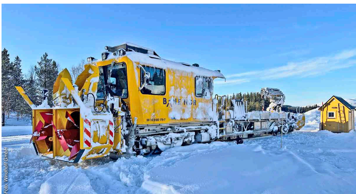
Gleisarbeitsfahrzeug MPV® VentuS® im Einsatz in Norwegen
